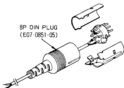
Fig. 9 8P DIN connector
